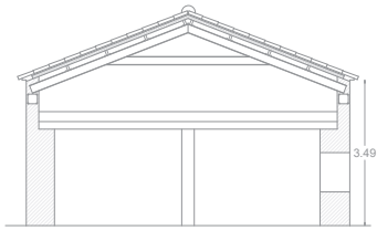
SECCIÓN TRANSVERSAL
